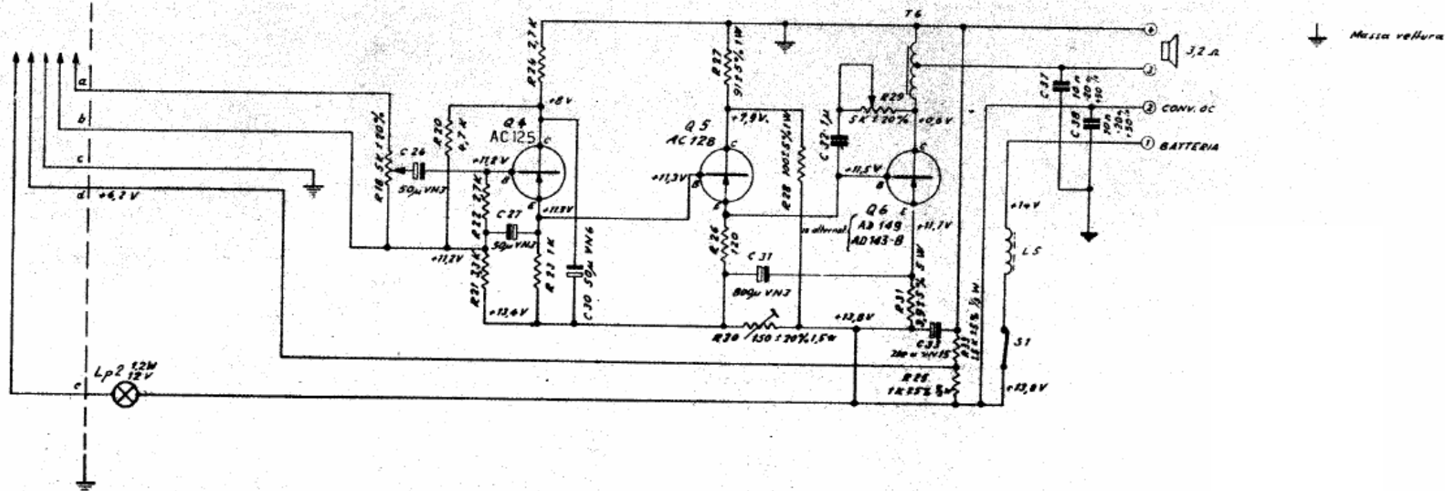
Schema elettrico della autoradio EA441A ed EA441A-L
